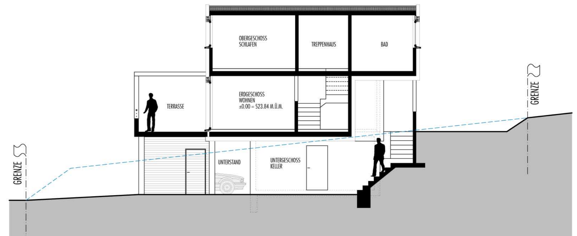
QUERSCHNITT
